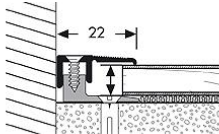
Abschluss-Profil
