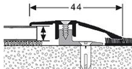
Anpassungs-Profil
