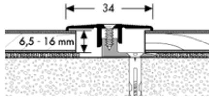
Übergangs-Profil
